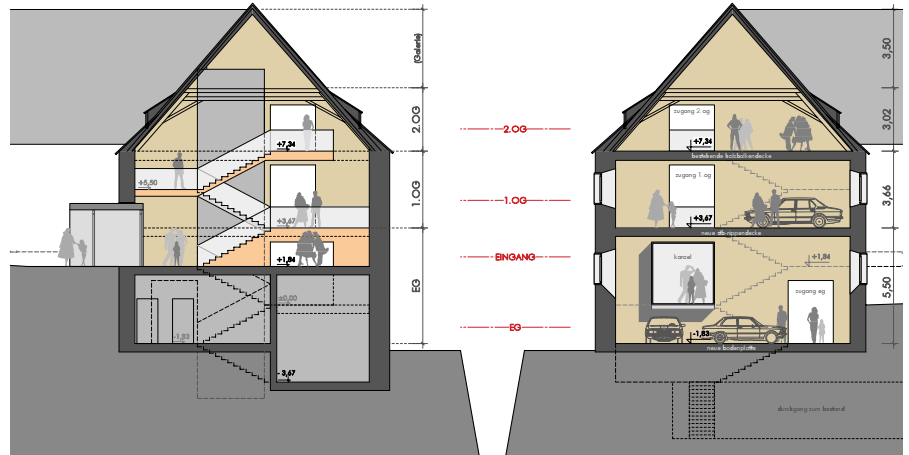
Schnitt durch den ehemaligen „Getreidekasten“
