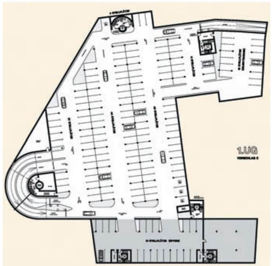
Das 1. Untergeschoss der „Tiefgarage Altstadt“
